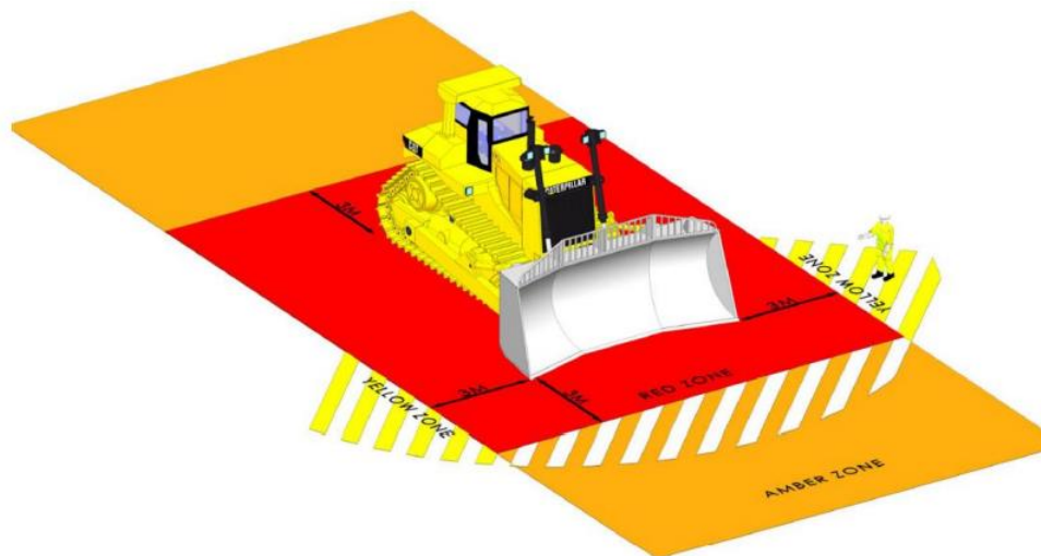
Gambar 13. Zona Keselamatan Bulldozer
