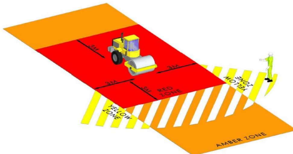
Gambar 20. Zona Keselamatan Tandem roller
