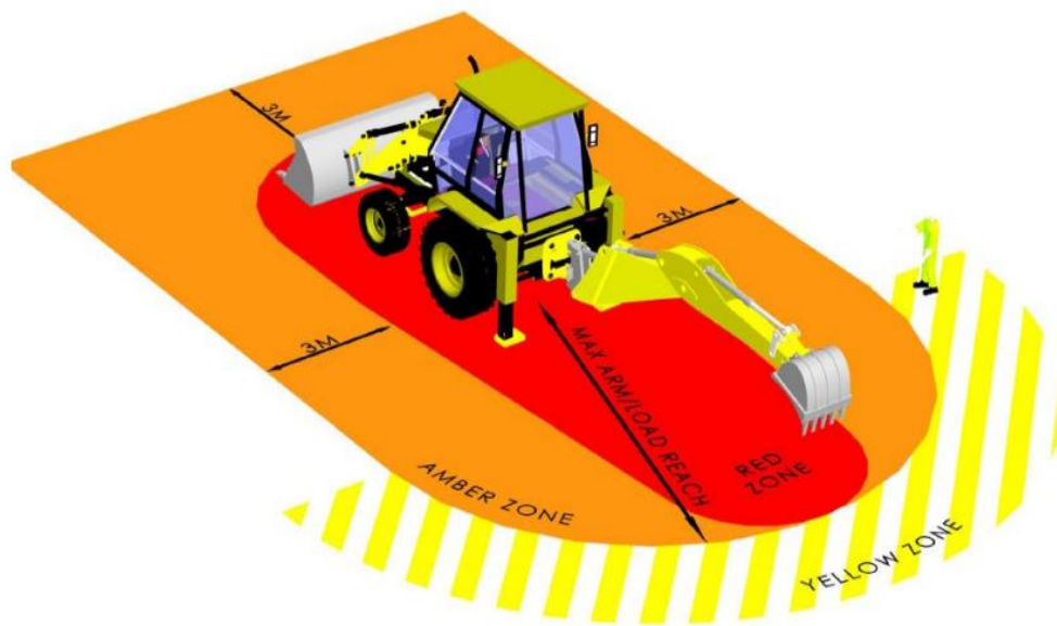
Gambar 11. Zona Keselamatan Backhoe
